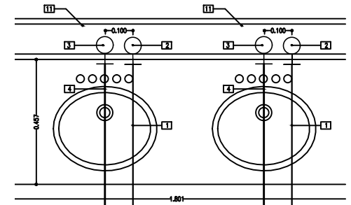
PLANTA LAVAMANOS DOBLE INFANTIL ESCALA 1:10
