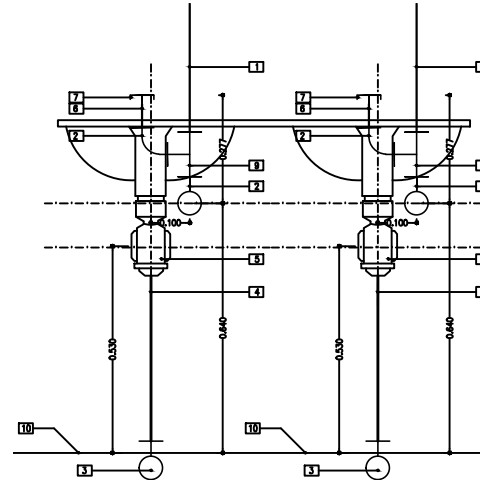
VISTA FRONTAL LAVAMANOS DOBLE INFANTIL ESCALA 1:10
