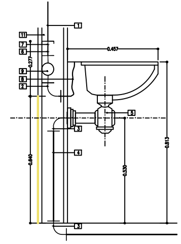
VISTA LATERAL LAVAMANOS DOBLE INFANTIL ESCALA 1:10
