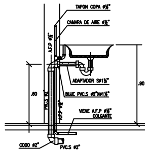
PLANTA CARCAMO DE DESAGUES ESCALA 1:10
