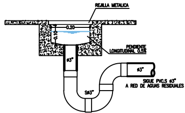
PLANTA CARCAMO DE DESAGUES ESCALA 1:10
