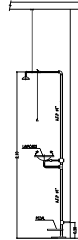
VISTA LATERAL LAVAJOS ESCALA 1:20
