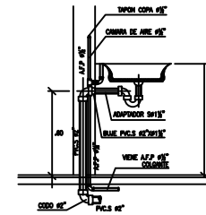
VISTA LATERAL LAVAMANOS ESCALA 1:20
