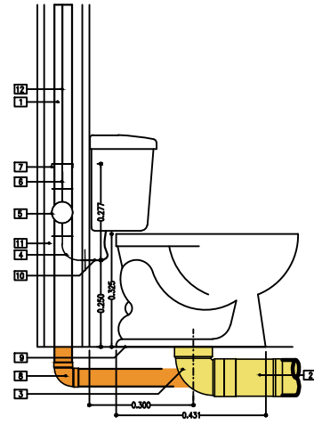
VISTA LATERAL SANITARIO TANQUE INFANTIL ESCALA 1:10
